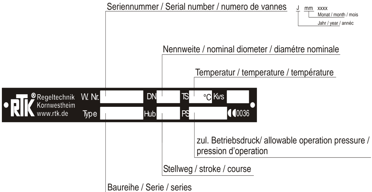
Bild 1/ Figure 1 : Typenschild auf Ventil / nameplate on valves /
